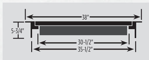
DOOR DIMENSIONS - TOP VIEW
