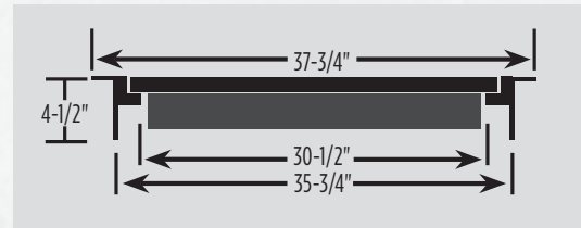
DOOR DIMENSIONS - TOP VIEW
