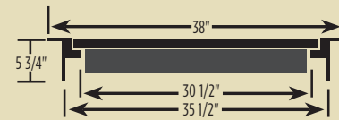
DOOR DIMENSIONS - TOP VIEW
