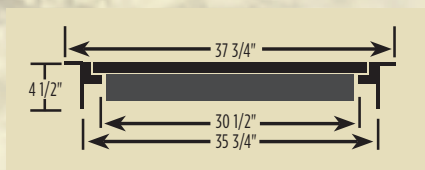
DOOR DIMENSIONS - TOP VIEW
